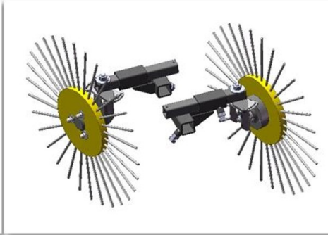
Doppelflachhäufler für Getreide bis 25 und 30 cm
