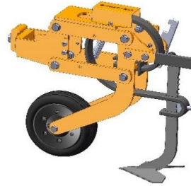
Einzel Parallelogramm - EPP
