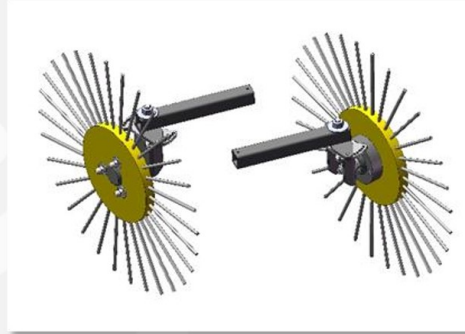
Nachlaufstriegel für Kombi-Parallelogramm
